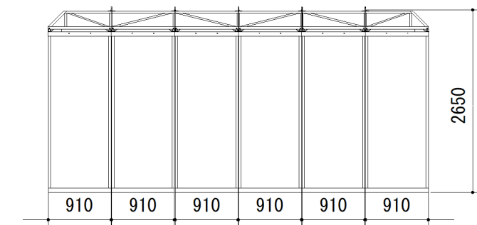
B立面図 S=1:75
