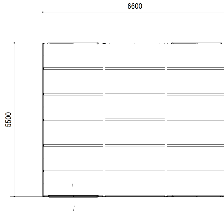
平面図 S=1:75
