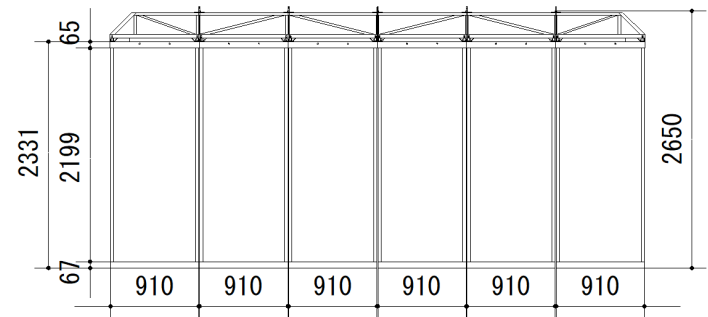
D立面図 S=1:75
