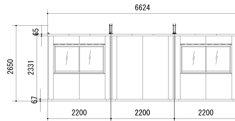
A立面図 S=1:75
