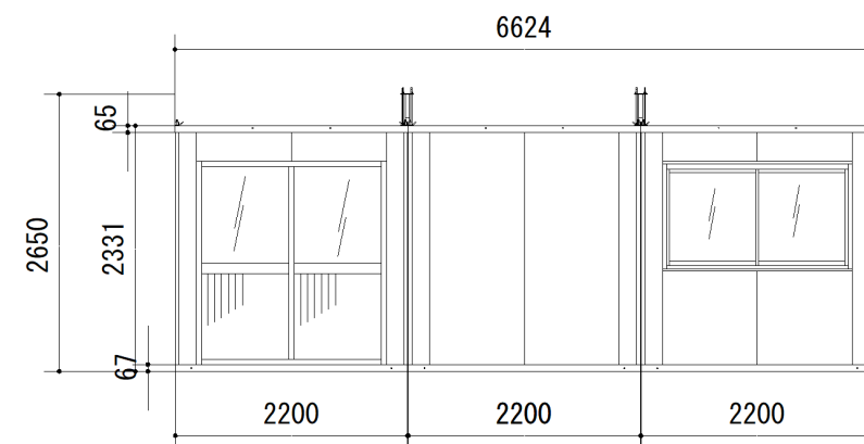
C立面図 S=1:75
